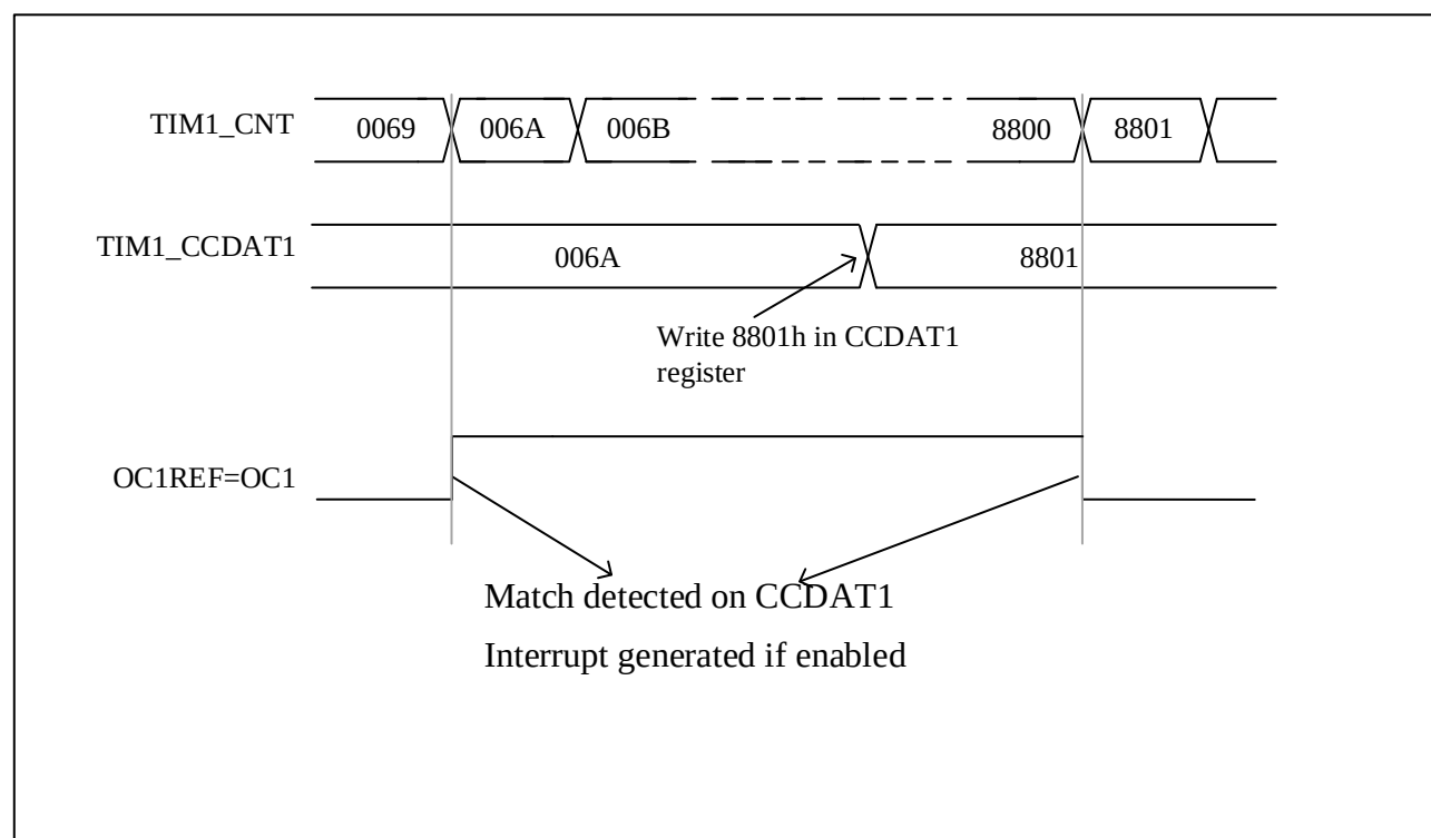
图 11-21 输出比较模式，开启 OC1
