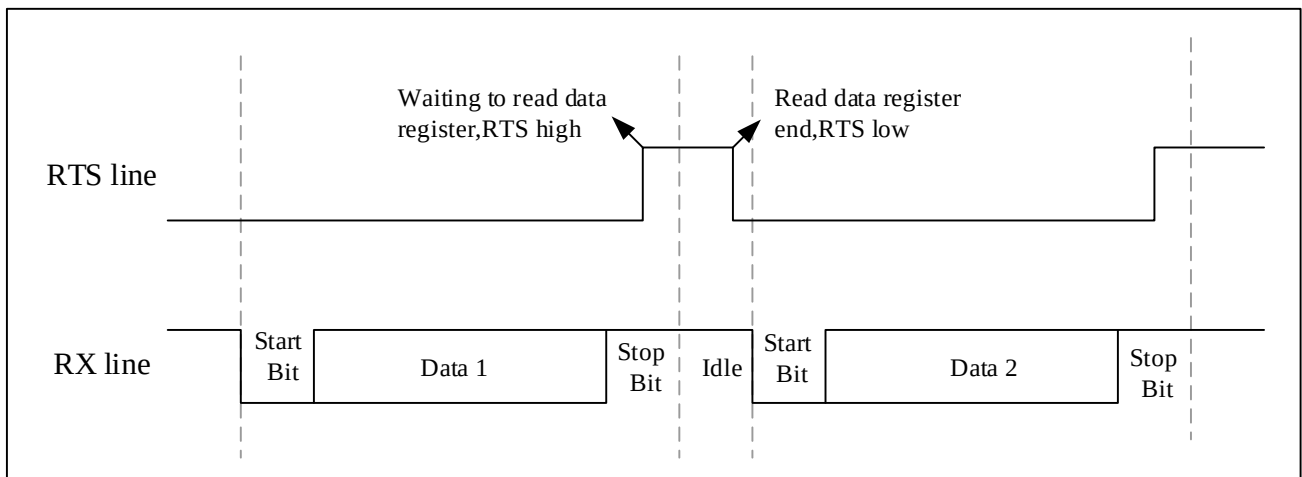
图 23-11 RTS 流控制
