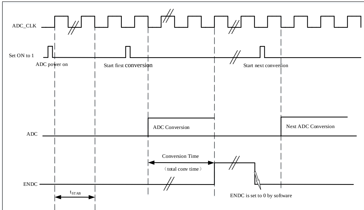
图 9-4 时序图
