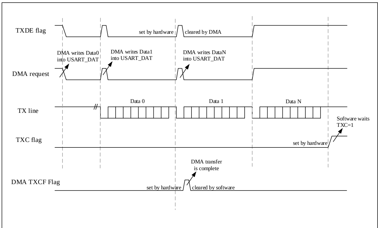
图 23-8 DMA 发送
