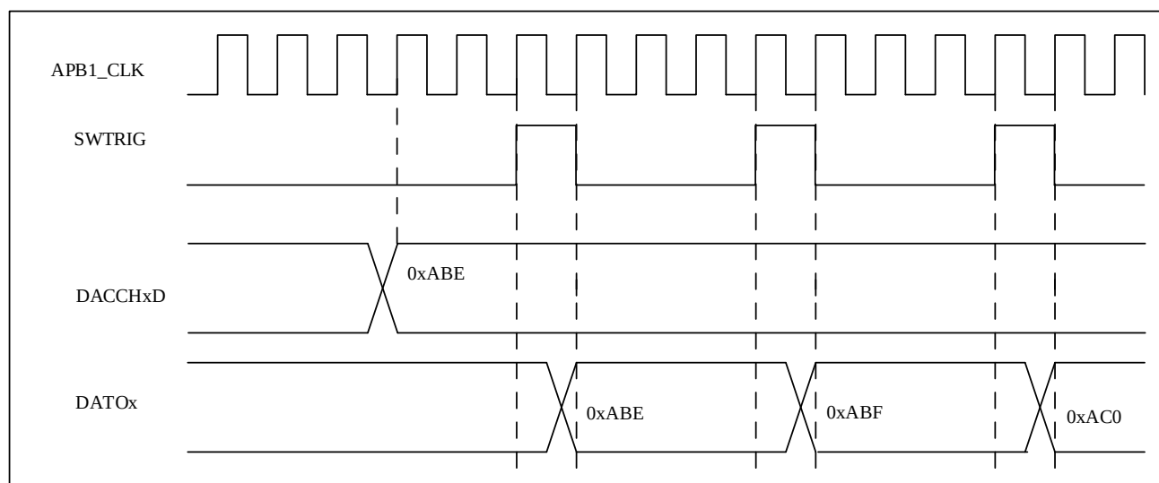
图 10-8 带三角生成的 DAC 转换（使能软件触发）
