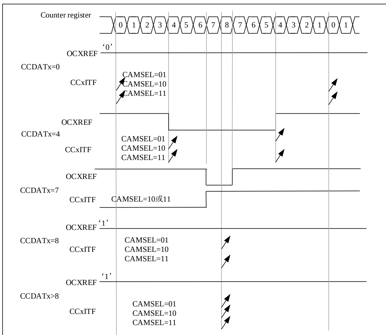
图 11-22 中央对齐的 PWM 波形 (AR=8)
