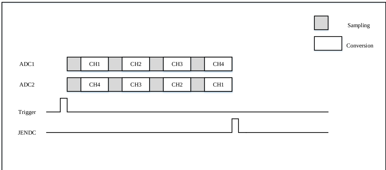
图 9-9 4 个通道的同步注入模式转换示意图
