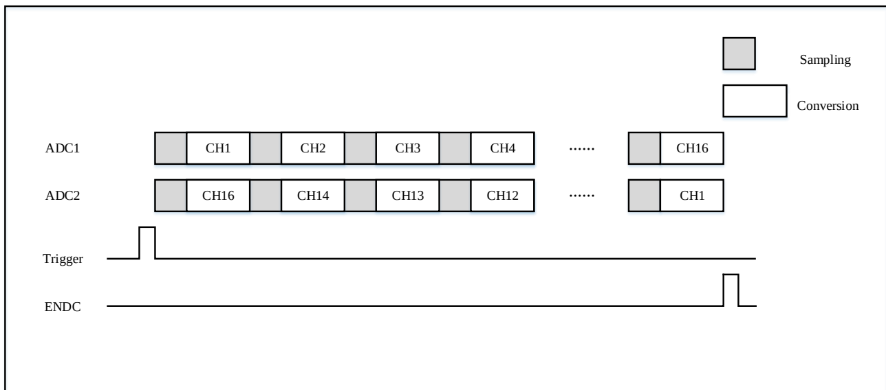
图 9-8 16 个通道的同步规则模式转换示意图
