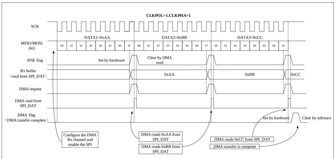
图 21-12 使用 DMA 接收
