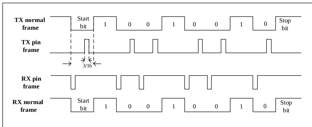
图 23-20 IrDA 数据调制 (3/16)-正常模式
