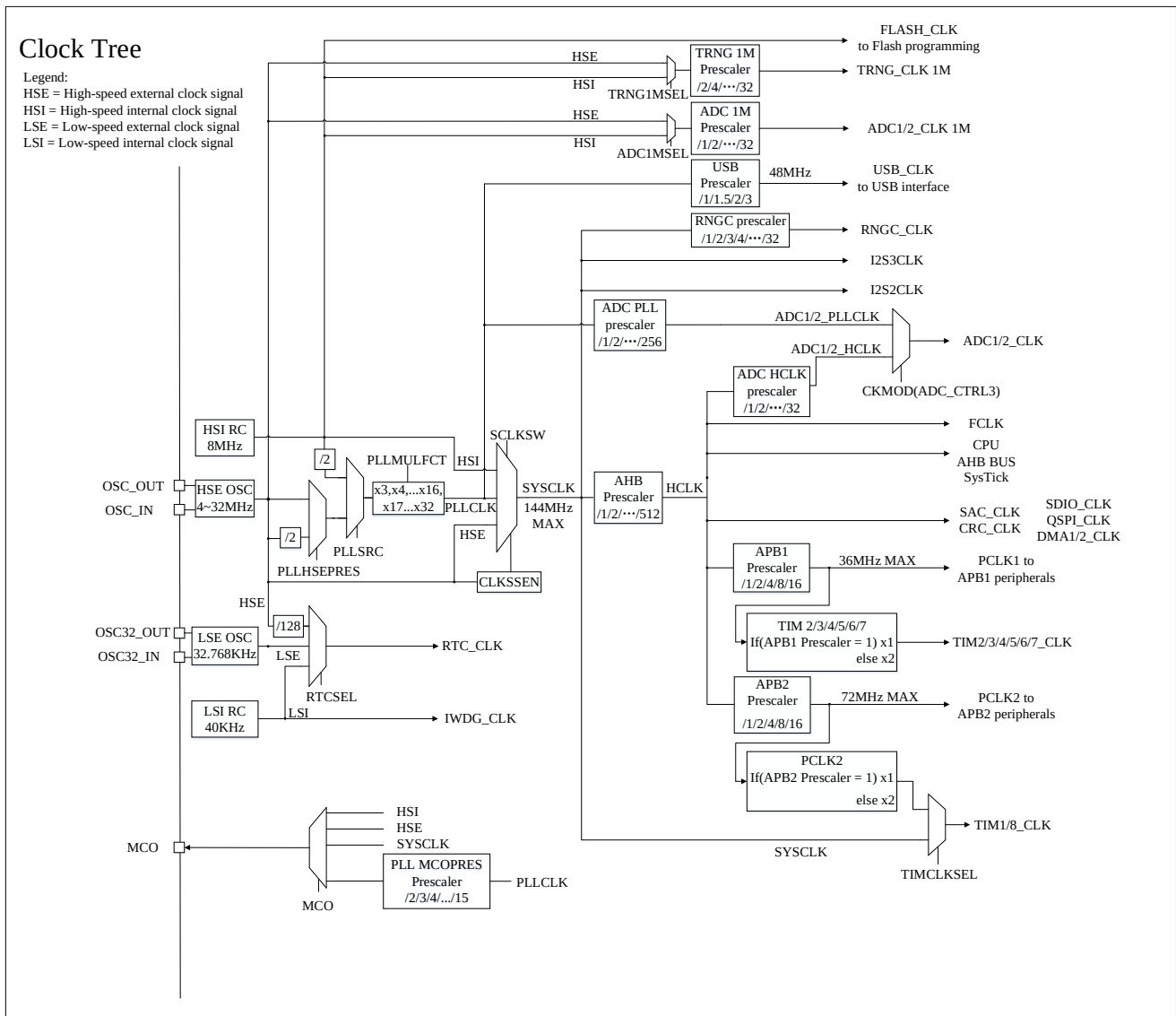
图 5-2 时钟树
