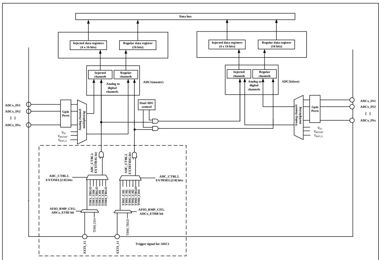
图 9-7 双 ADC 框图
