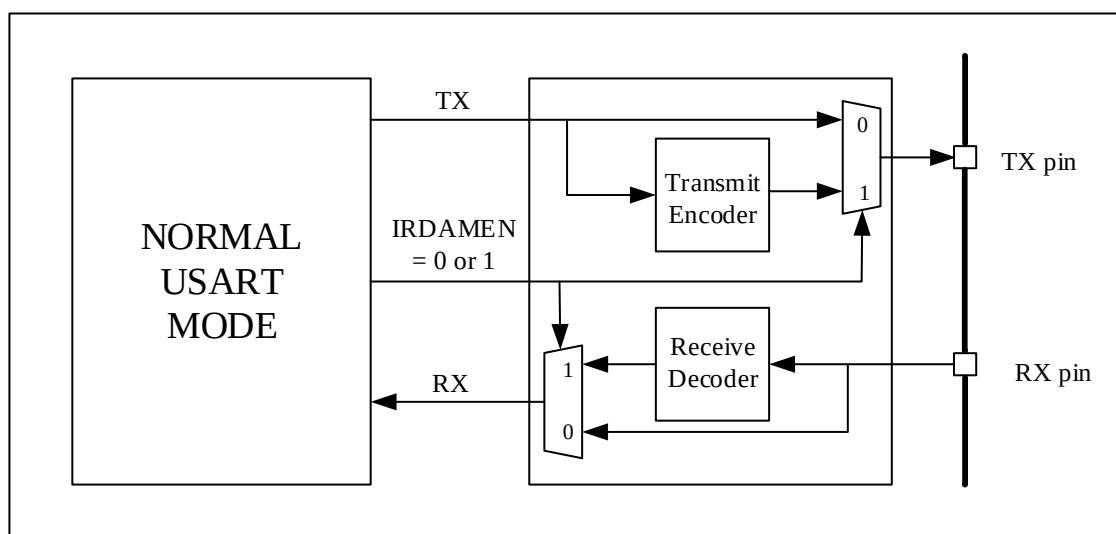
图 23-20 IrDA 数据调制 (3/16)-正常模式
