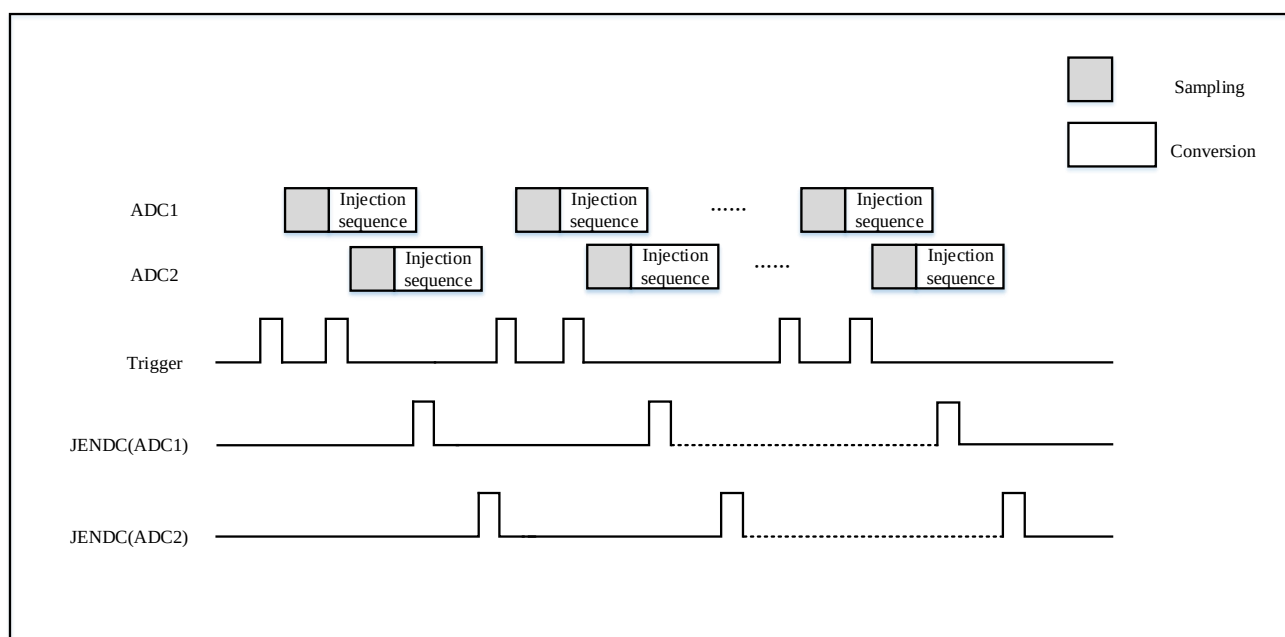
图 9-12 交替触发：注入通道组
