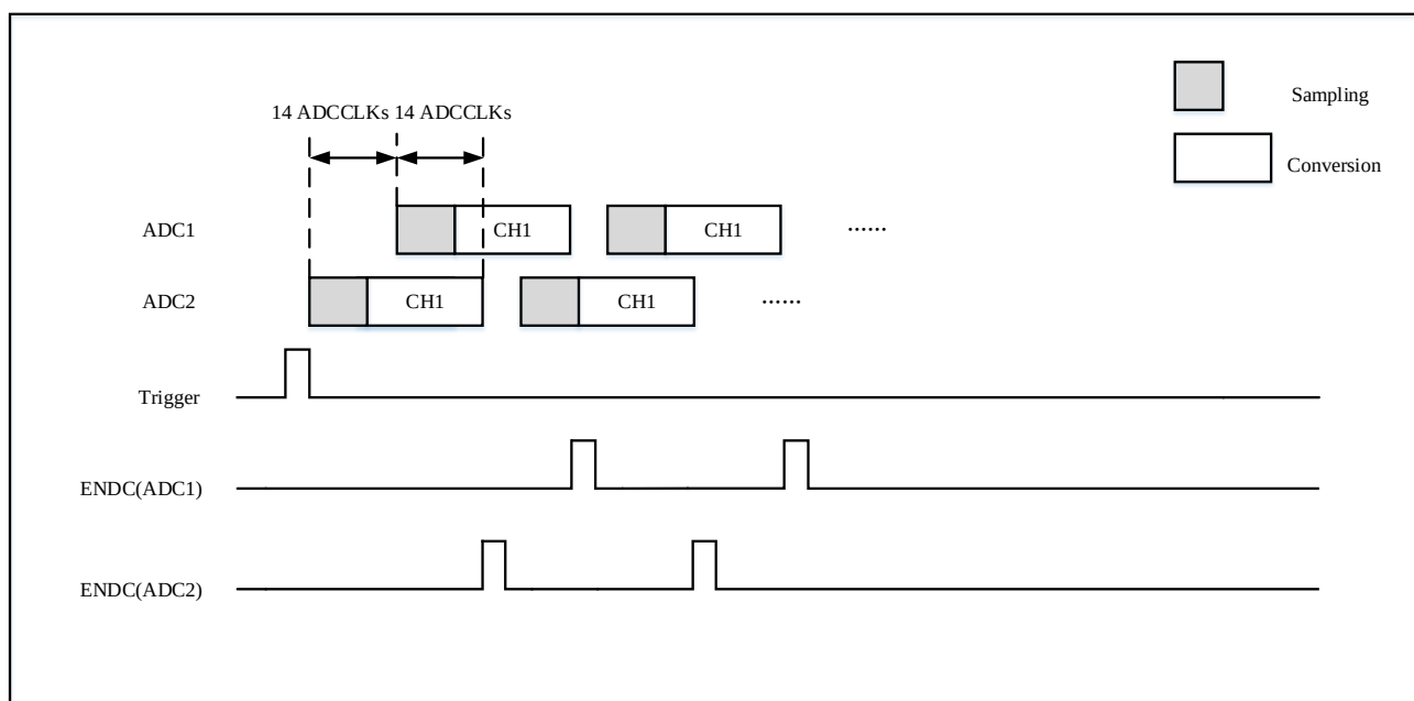
图 9-11 1 个通道的慢速交叉模式转换示意图
