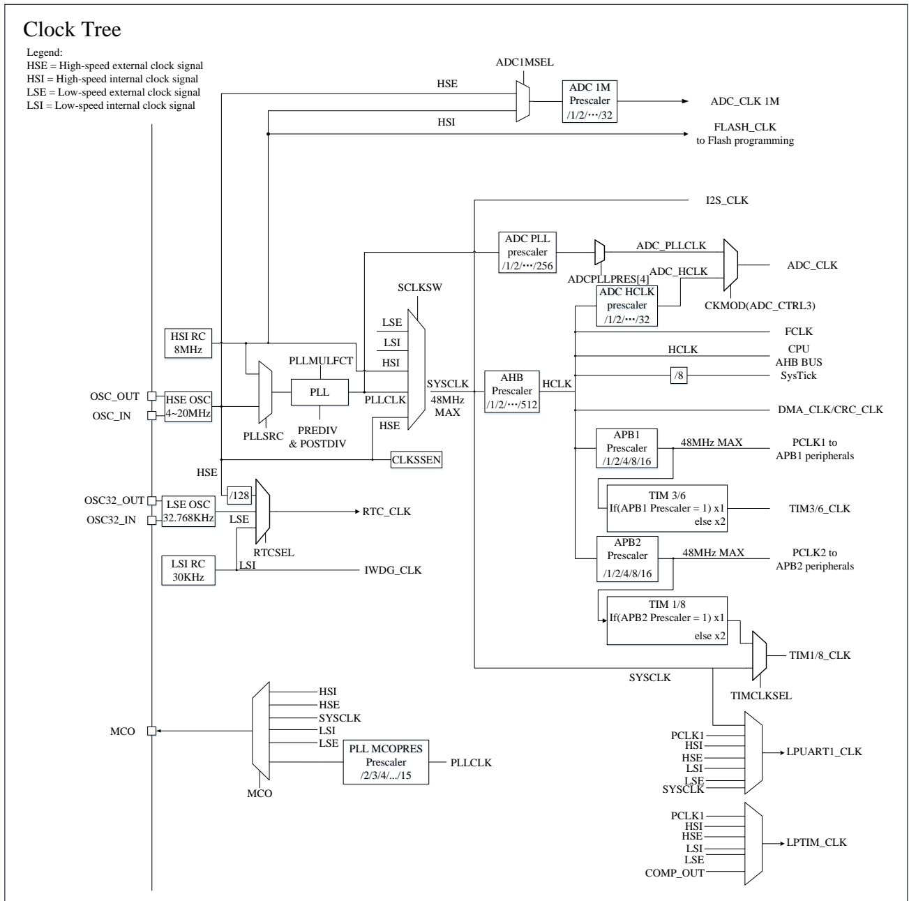
图 4-2 时钟树
