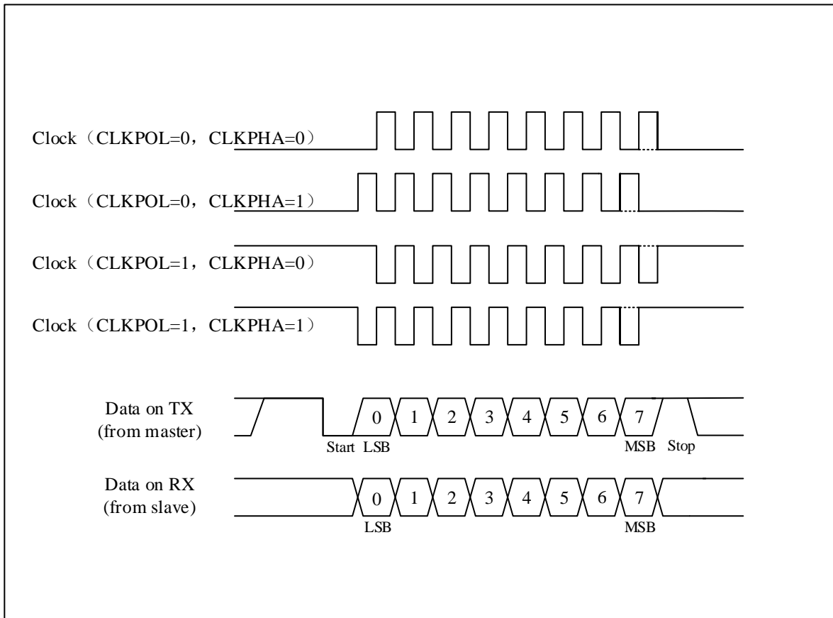
图 18-16 USART 数据时钟时序示例 (WL=0)
