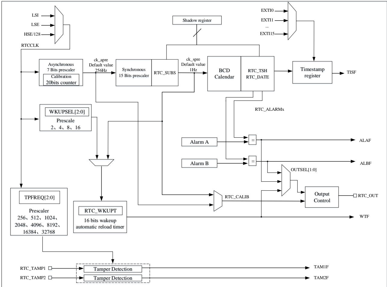
图 21-1 RTC 框图
