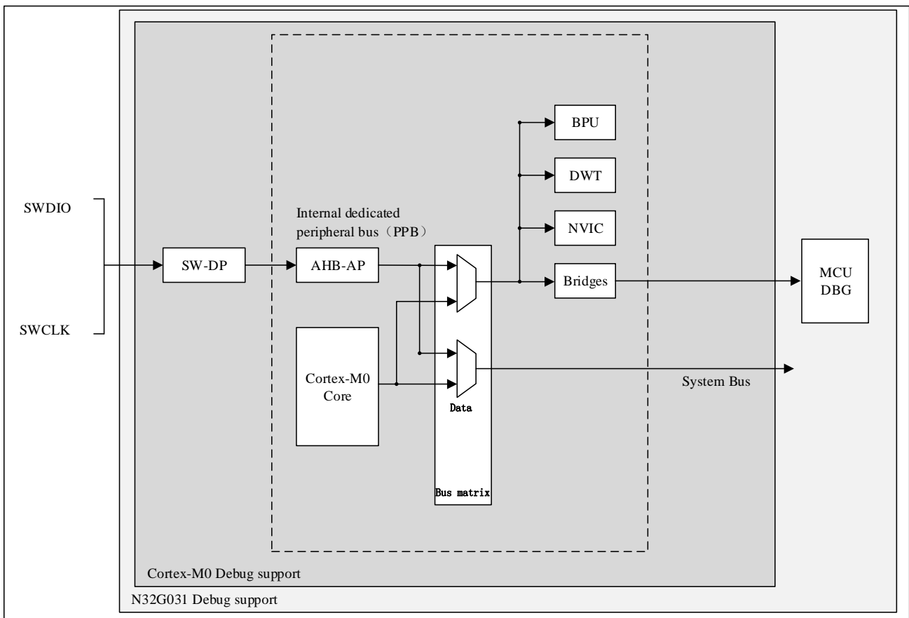
图 25-1 N32G031 级别和 Cortex ® -M0 级别的调试框图
