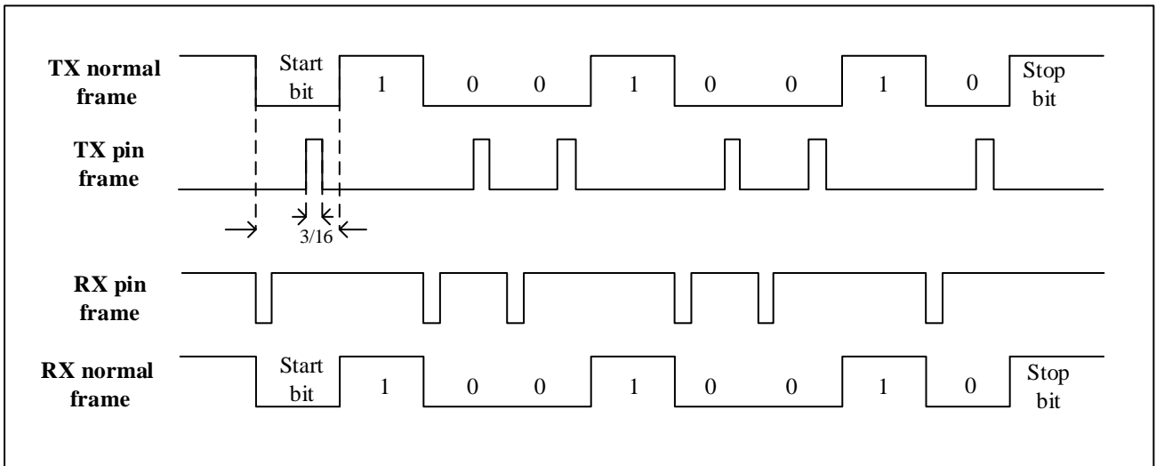
图 18-20 IrDA 数据调制(3/16)-正常模式
