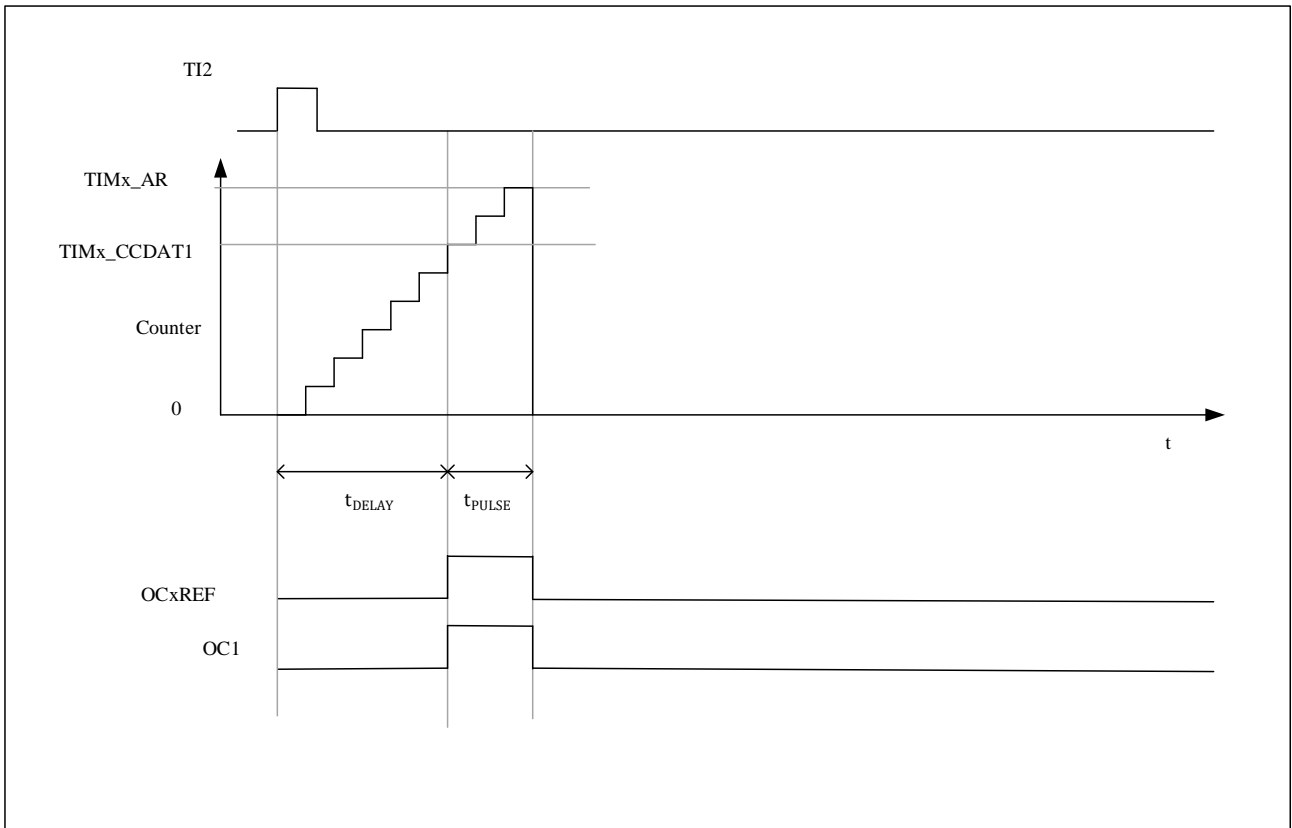
图 10-20 单脉冲模式示例
