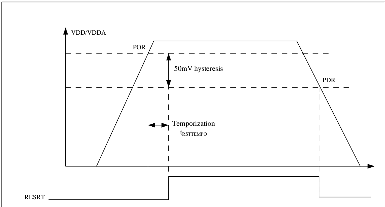
图 3-2 上电复位和掉电复位的波形图
