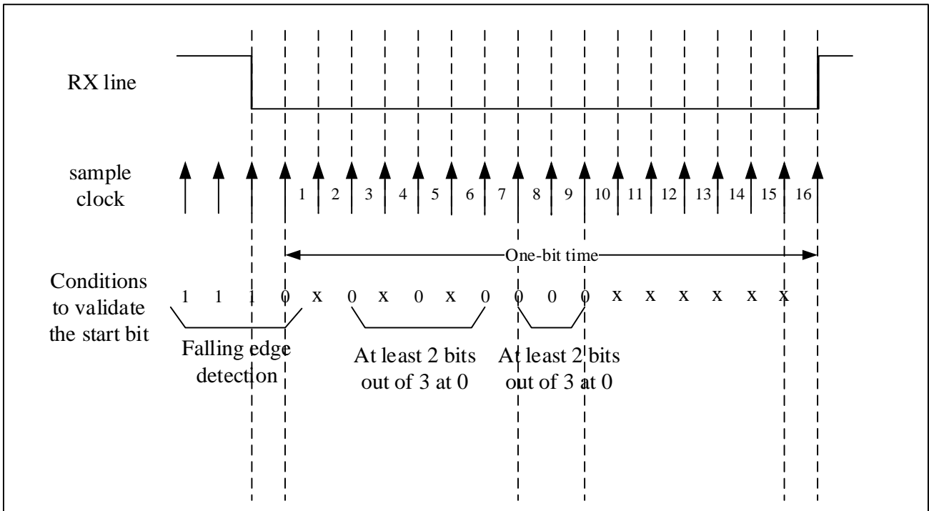
图 18-7 起始位检测
