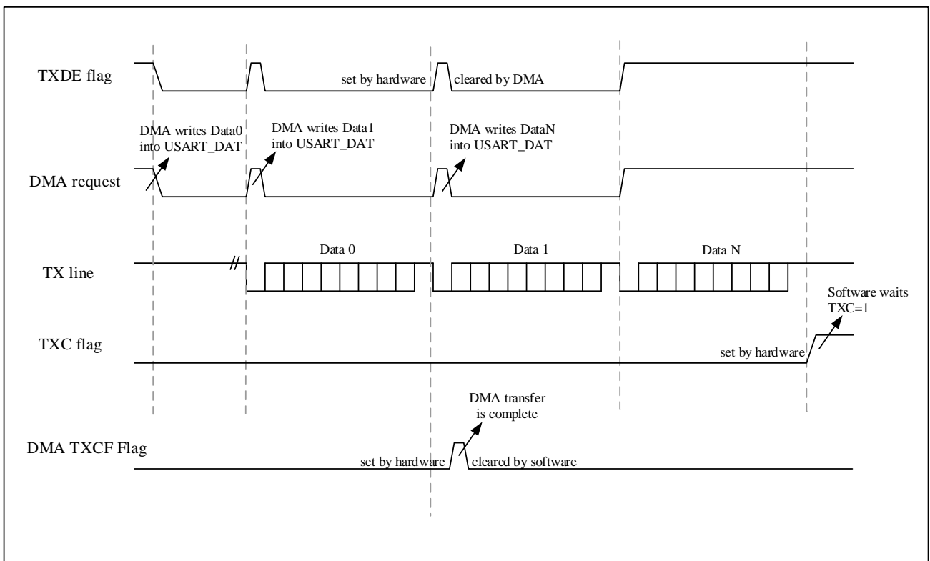
图 18-8 DMA 发送
