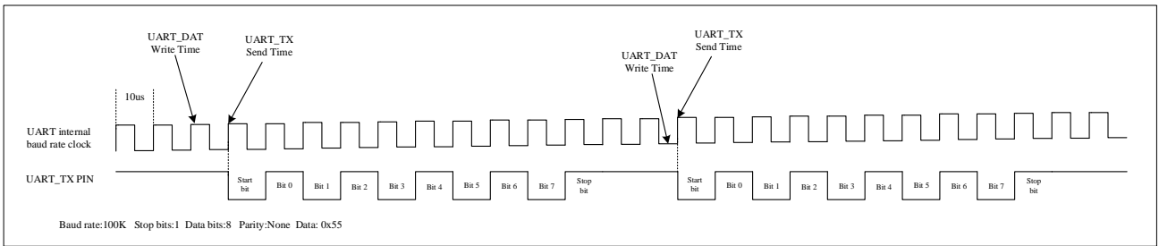
图 18-5 发送时差
