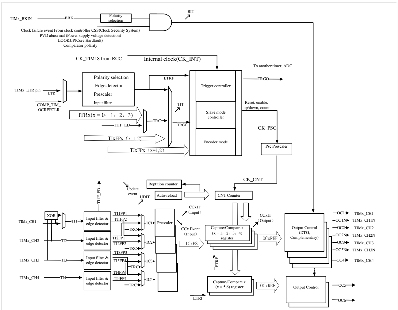
图 9-1 TIMx(x=1/8)框图
