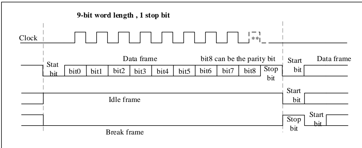
图 18-3 字长=9 设置
