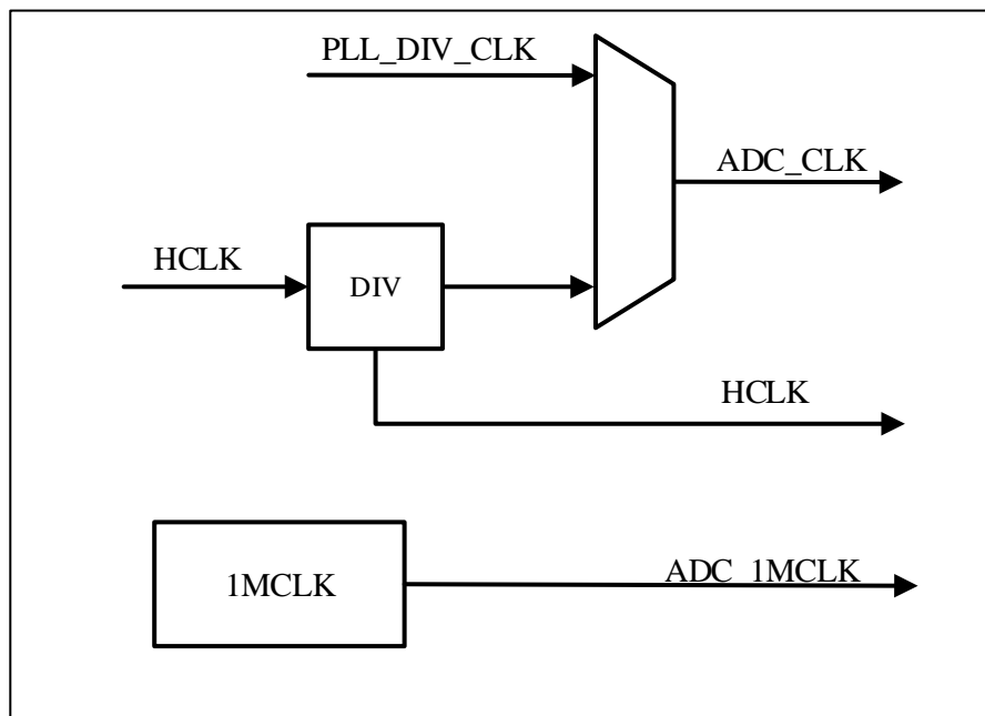
图 15-2 ADC 时钟
