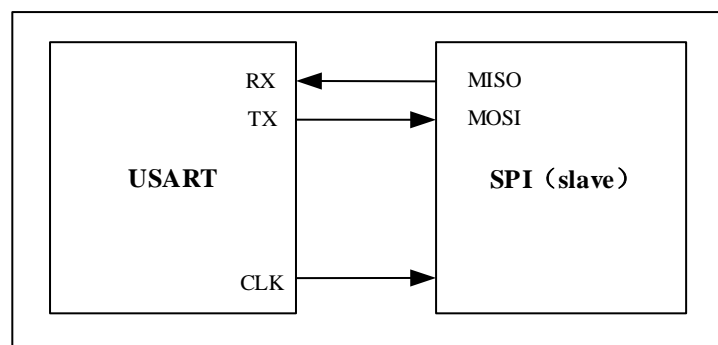
图 18-15 USART 同步传输示例
