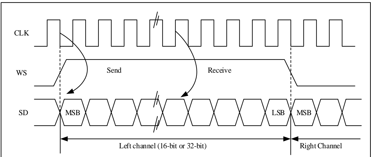
图 20-17 MSB 对齐 16 位或 32 位全精度，CLKPOL = 0
