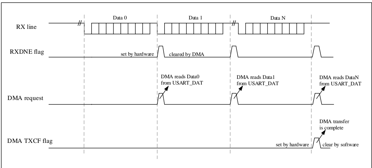
图 18-9 DMA 接收
