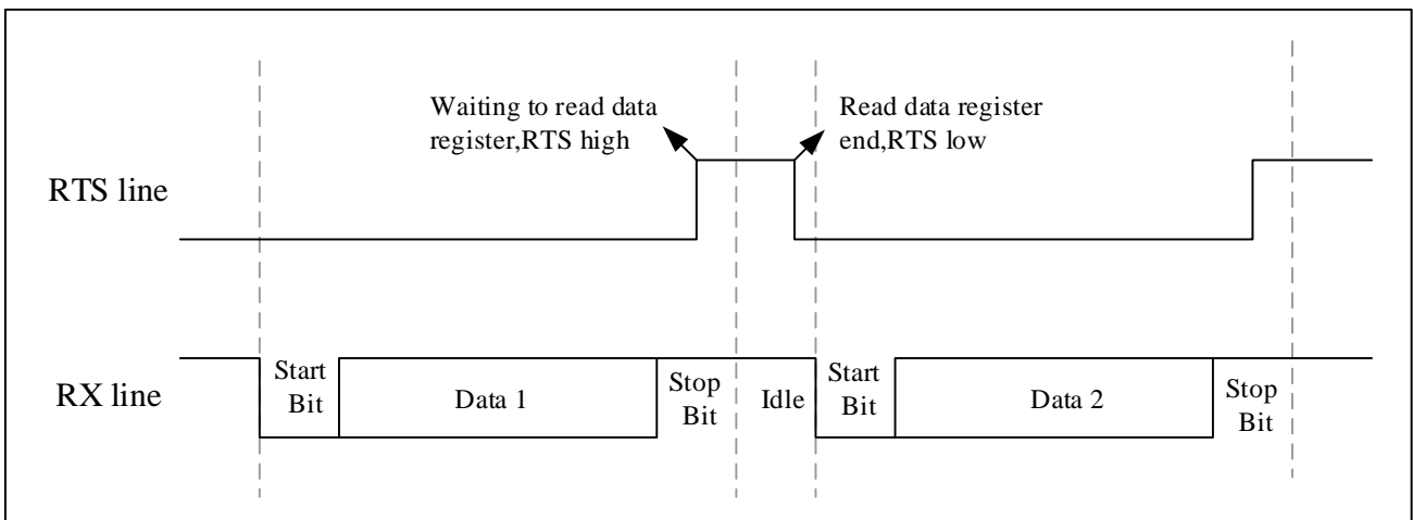
图 18-11 RTS 流控制
