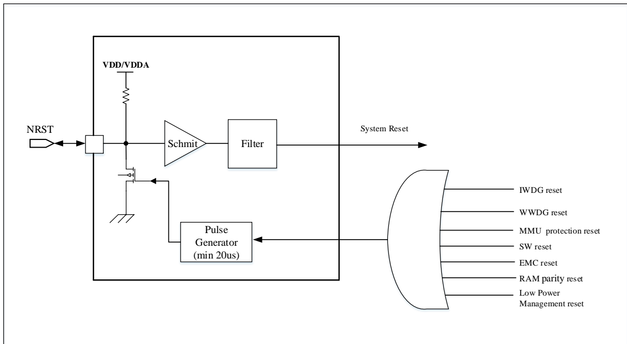
图 4-1 复位电路
