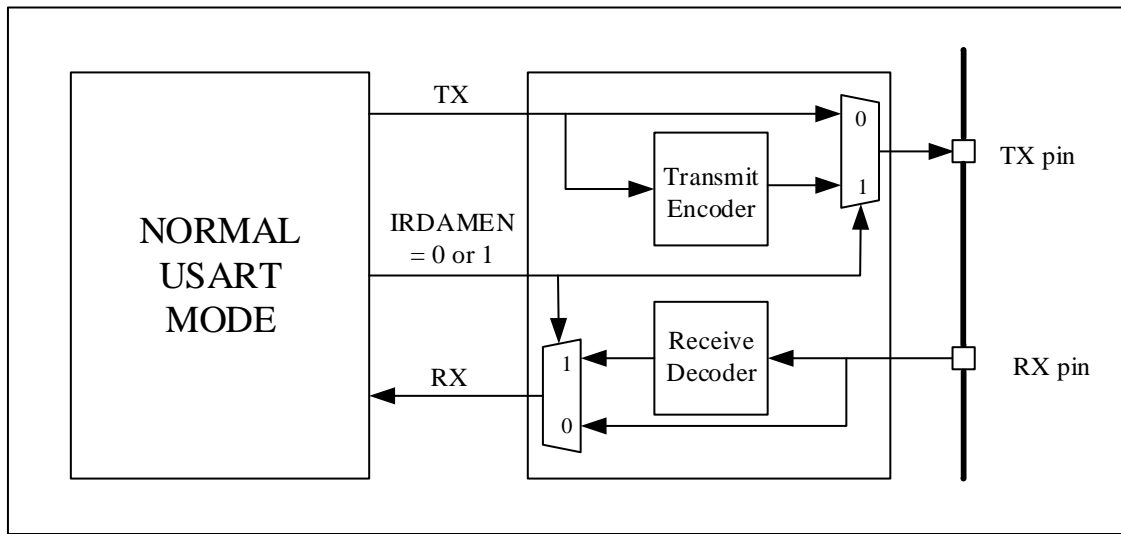
图 18-20 IrDA 数据调制(3/16)-正常模式
